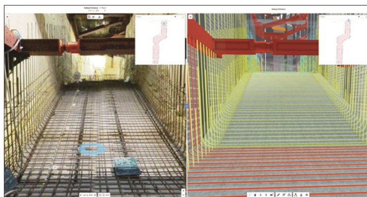
現場(左)と BIM モデル(右)の配筋を同じ視点で比較
